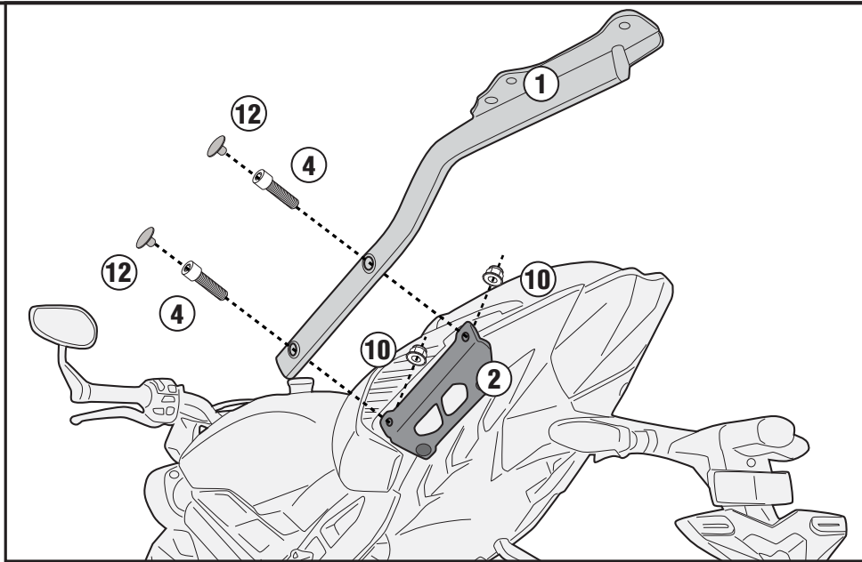
M5 PLATE
