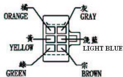
"A" 詳圖
